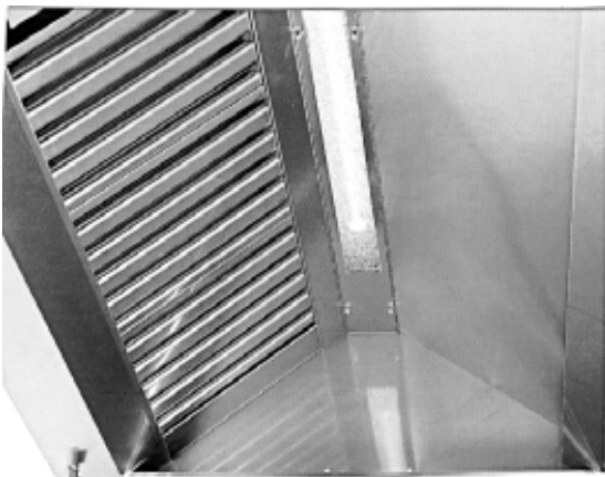
26 - DÉTAIL DE L'ÉCLAIRAGE EN ENCASTRÉ
