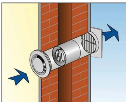
Traversée du mur directe
