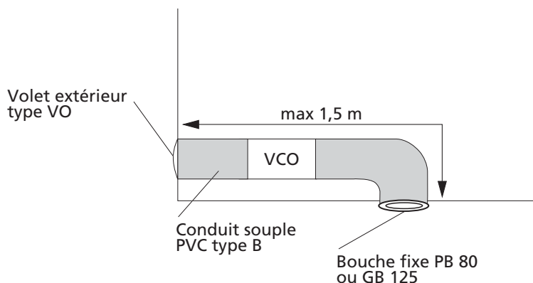
Raccordement à un conduit court.
